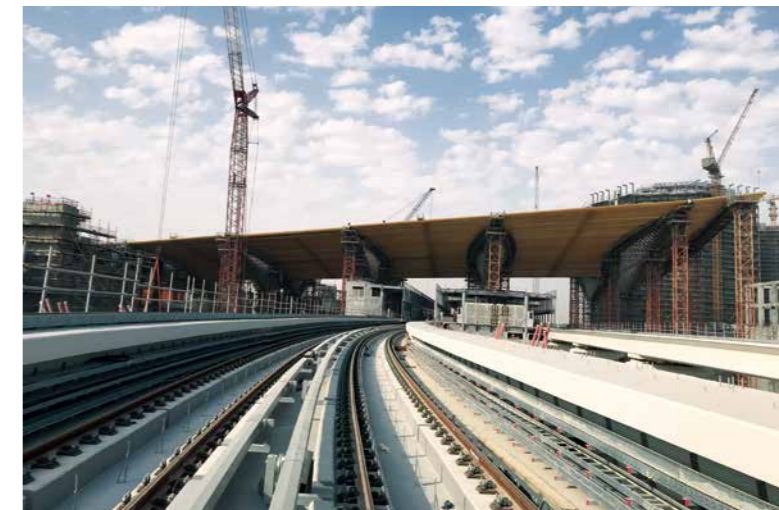
迪拜地铁世博站项目现场。
